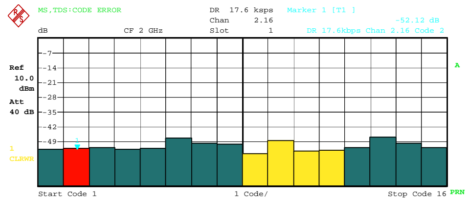
Bild 5-9 CDEP-Diagramm
