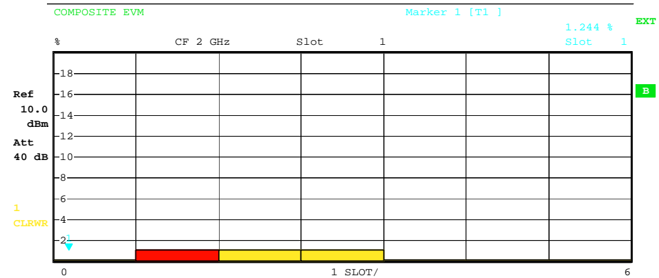
Bild 5-10 Composite-EVM-Diagramm
