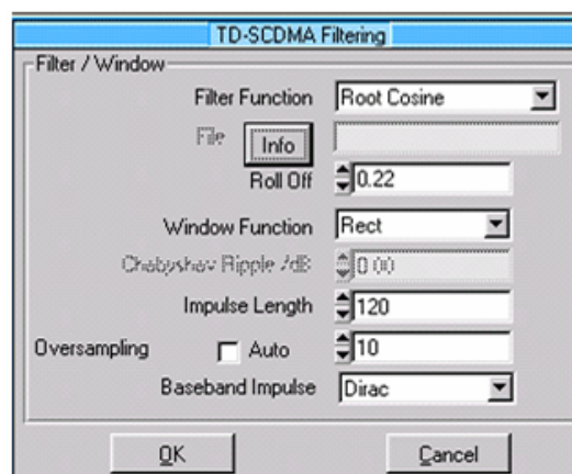
Bild 2-2 WinIQSIM – Sendefiltereinstellungen
