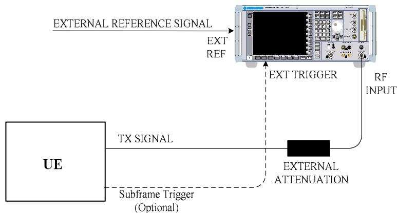
Bild 3-1 MS-Messaufbau
