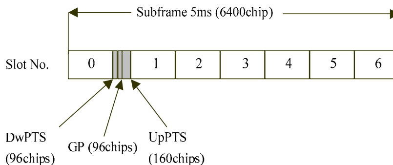
Bild 2-6 Subframe-Struktur
