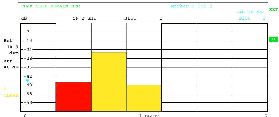
Bild 5-13 Peak-Code-Domain-Error-Diagramm bei nicht erkannten Kanälen.
