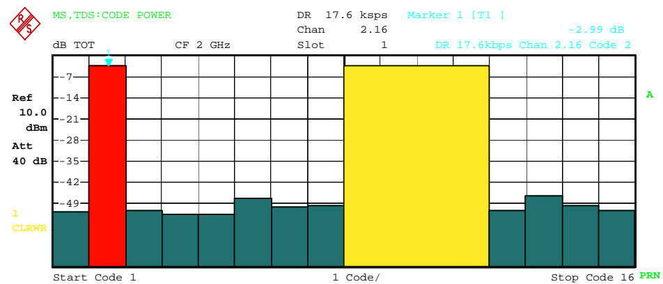
Bild 5-8 CDP-Diagramm
